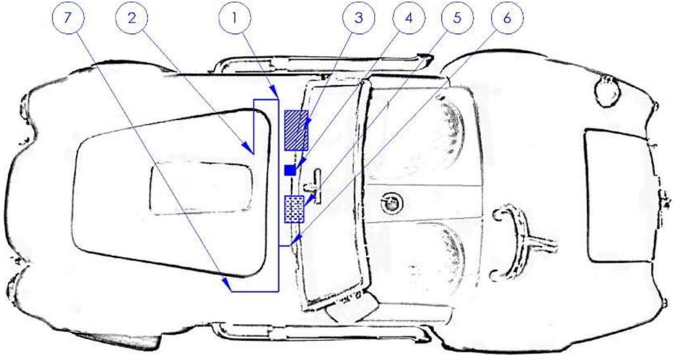
2011-2014 wiring layout
